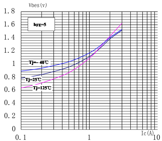
V_{bes} - I_c
