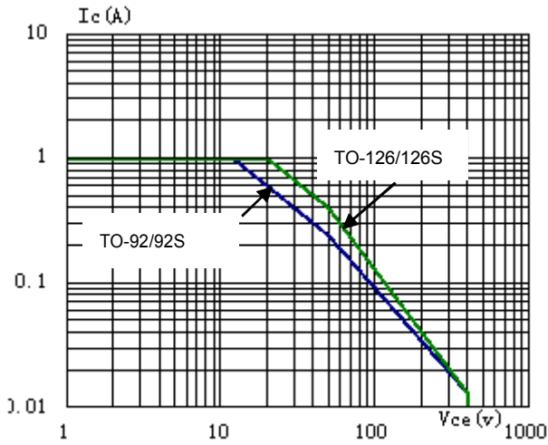
SOA (DC)
