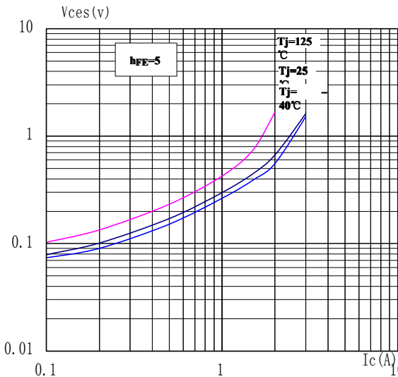
V_{ces} - I_c
