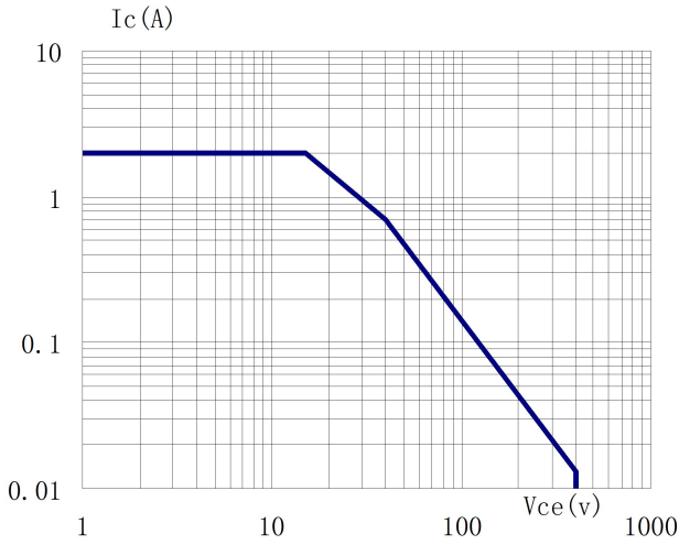
SOA (DC)
