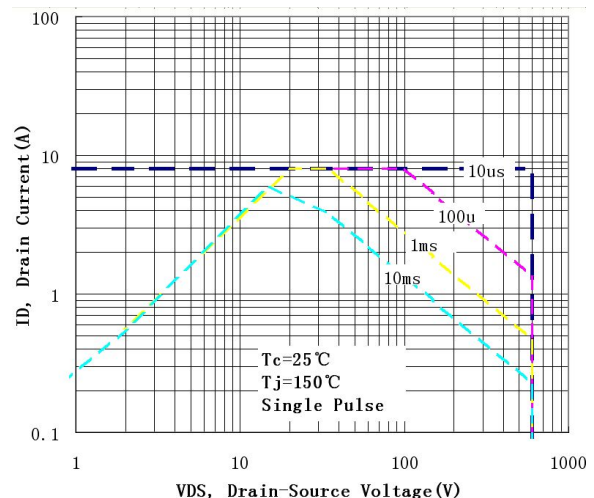
图 6 最大安全工作区曲线
