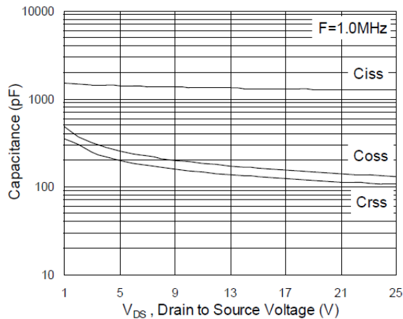
图 5 电容曲线
