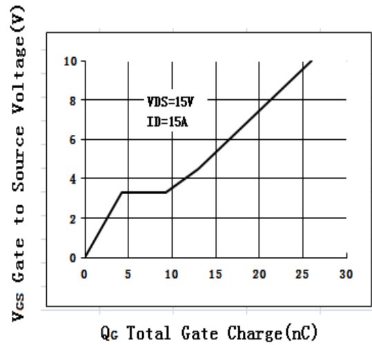
图 4 栅电荷波形
