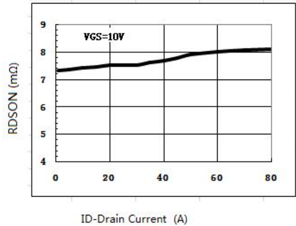
图 2 导通电阻与漏极电流的曲线
