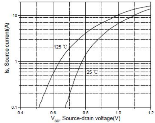
图 2 二极管正向电压曲线 Fig2 Typical Source-Drain Diode Forward Voltage
