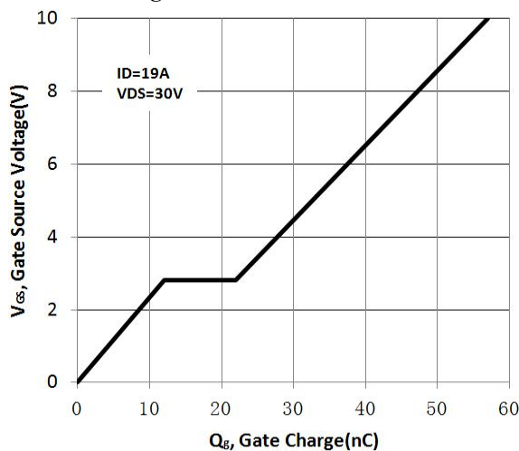
图 4 栅电荷波形
