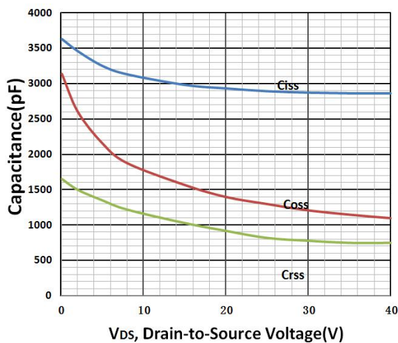
图 5 电容曲线
